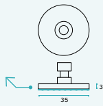
IN.08.BRG.35 Base de colar para toalheiro / Base to glue towel rack / Base para pegar toallero.
